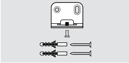
벽 장착 액세서리 장착 플레이트 부착 나사 맞춤못* 맞춤못 나사 *다양한 벽 유형에 따라 특정 맞춤못이 필요할 수 있습니다
